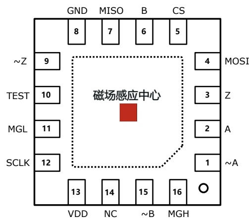
图 3: QFN-16L 3mmx3mm
