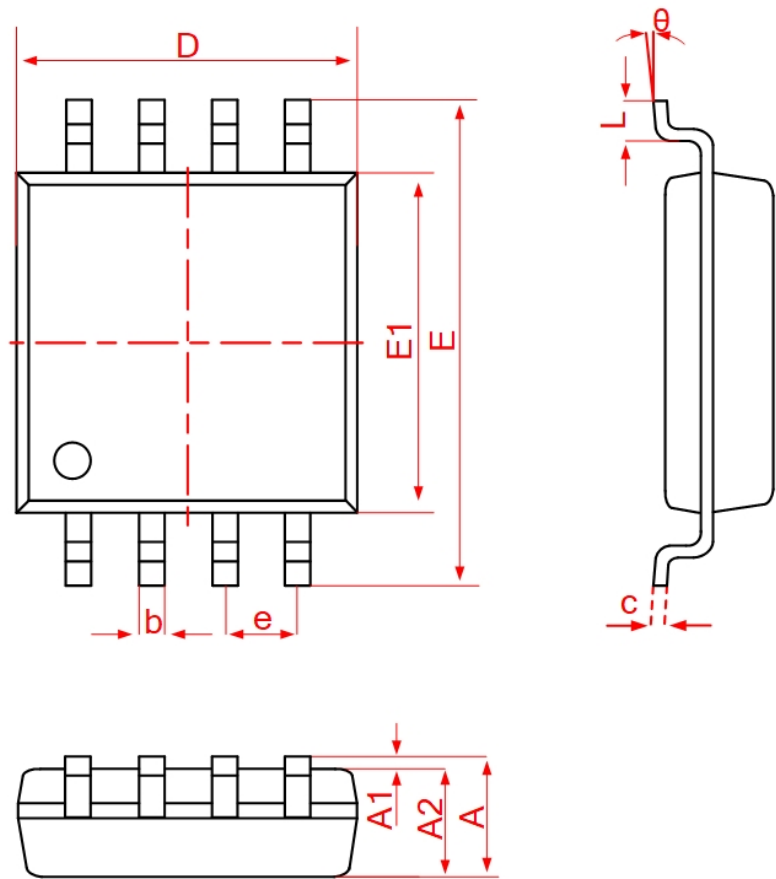
图 18: SOP-8 封装信息
