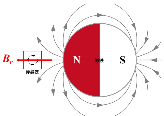
图 14: 传感器位于径向磁场示意图
