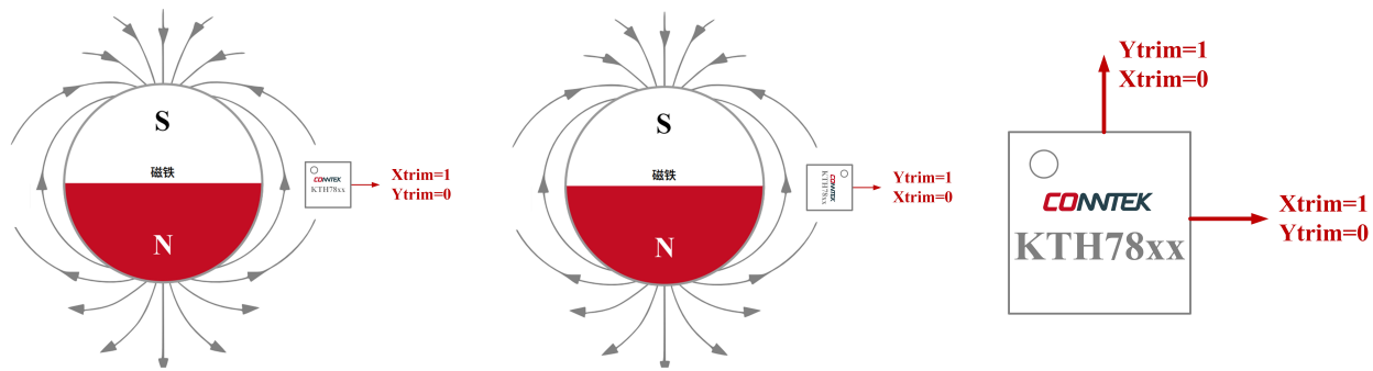
图 15: 芯片摆放方向与 Xtrim、Ytrim 参数的设置示意图
