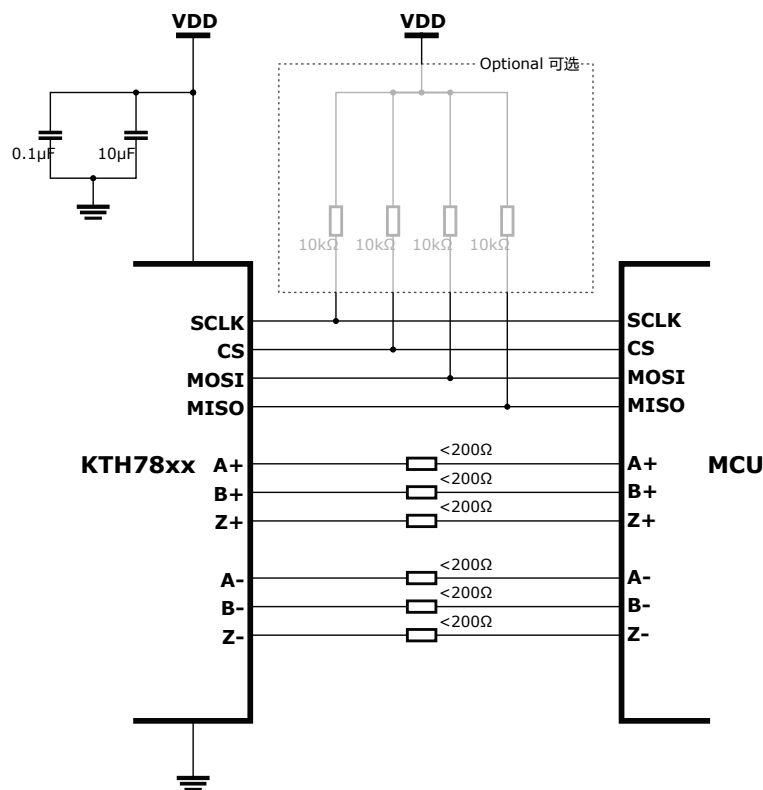
图 2: 应用电路
