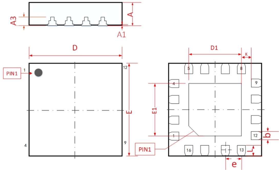
图 16: QFN-16L 封装信息
