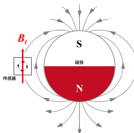
图 13: 传感器位于切向磁场示意图
