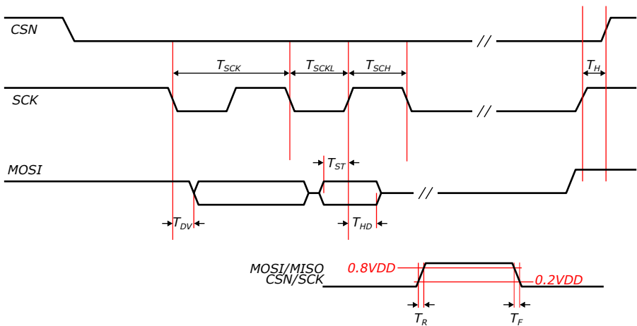
图 8: SPI 时序图
