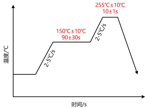
图 20: 焊接温度曲线
